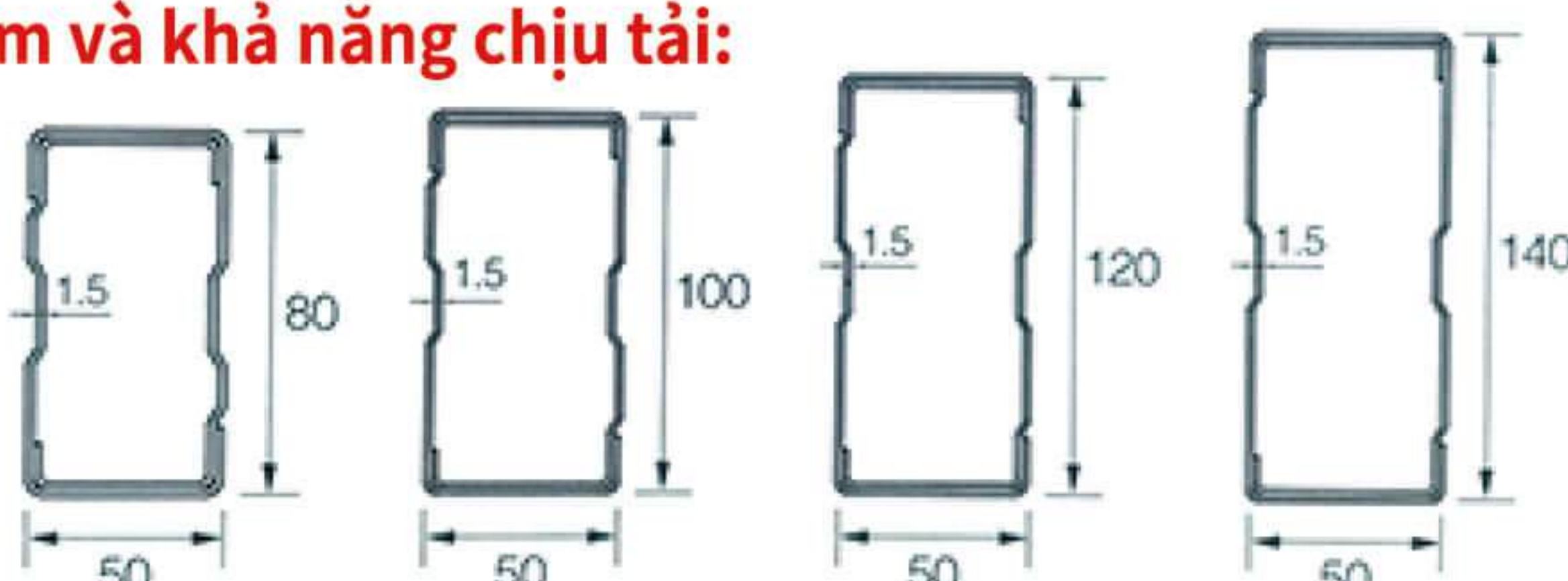
Các loại dầm hàn thường dùng
